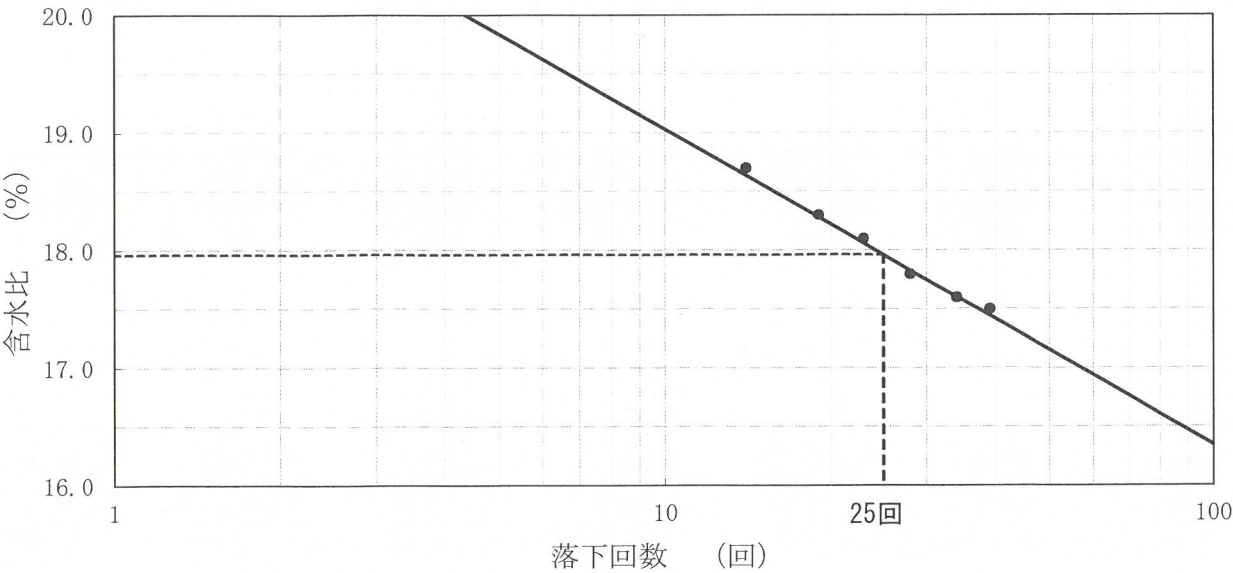
流動曲線
